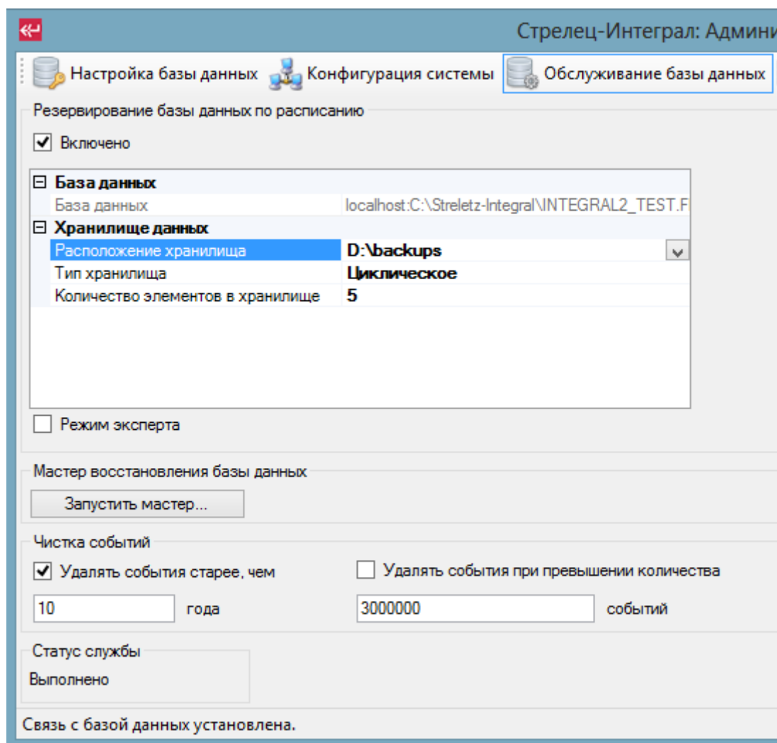
Рисунок 36 – Настройка обслуживания БД
